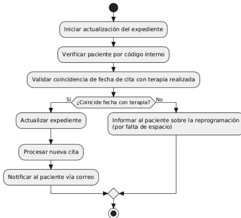
Caso 3: Diagrama de Actividades - Expediente del Paciente - Milton Gómez
