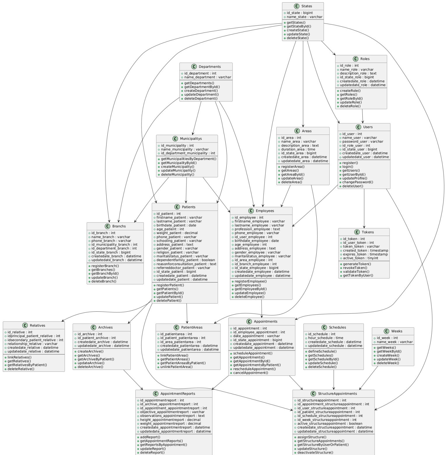
Diagrama de Clases - CADEP - Milton Gómez
